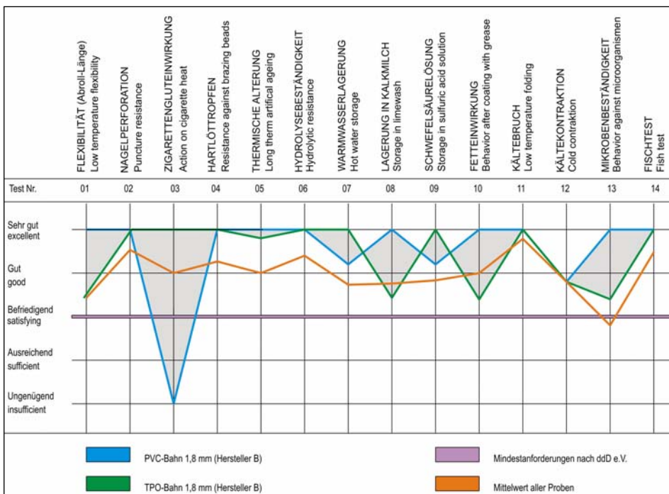
Darstellung 2: Verkleinerte Darstellung eines Eigenschaftsprofils für zwei 1,8 mm dicke Bahnen eines Herstellers im Vergleich:
